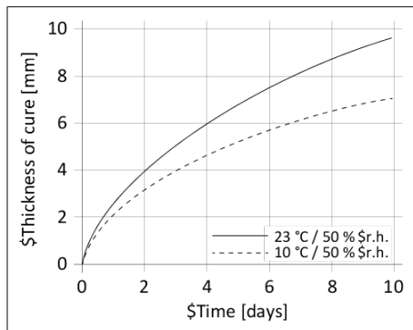
Diagramm 1: Durchhärtengeschwindigkeit Sikaflex®-508
